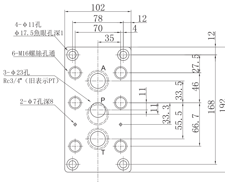
BUCG-06 安裝尺寸圖 Mounting Data
