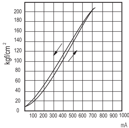
EBG-06(H)
