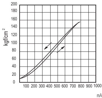
EBG-06(C)
