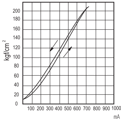
EBG-03(H)
