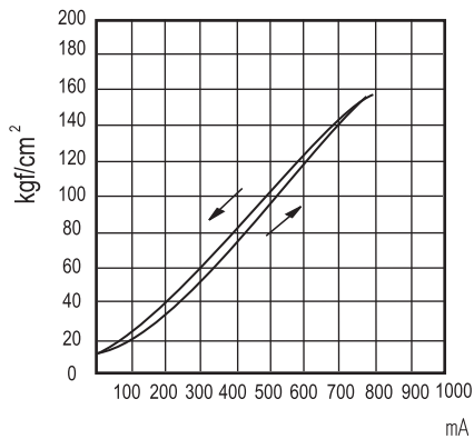
EBG-03(C)
