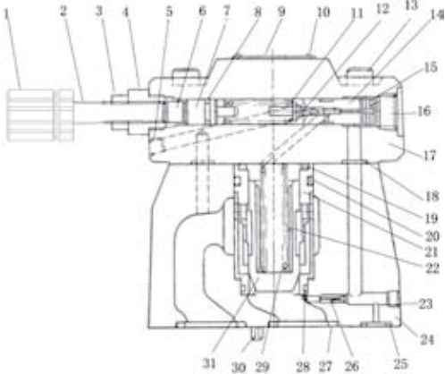
JRBS-G03/G06/G10 零件表 Psrat List
