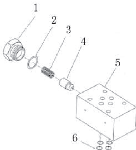
MC-02A/B/P/T 零件表 Psrat List
