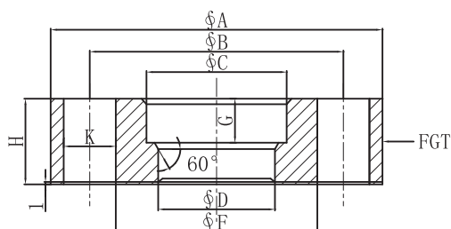
滿油閥 安裝法蘭參考尺寸 Flanges Dimensions(mm)
