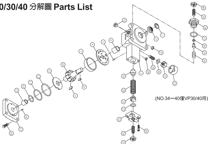
VP-15/20 零件表 Psrat List
